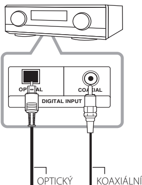
Zesilovač/Přijímač
